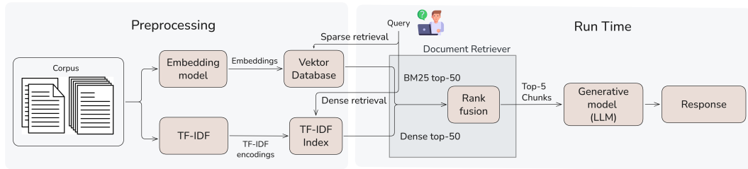
Gambar IV.3 Diagram Alur Pipeline Konfigurasi Baseline
