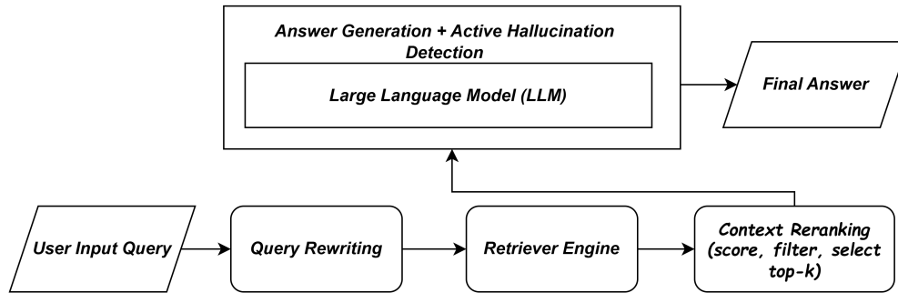
Gambar IV.1 Diagram alur sistem RAG-LLM untuk mitigasi halusinasi
